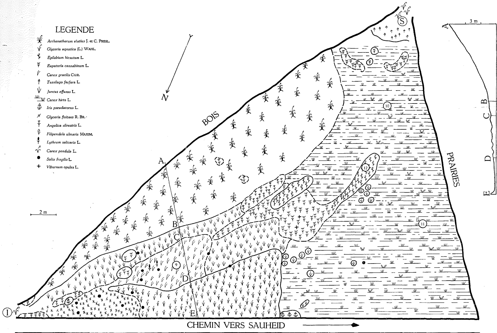
FIG. 3. — Limites et répartition des groupements végétaux. 9, 10, 11, 12 = aires des échantillons représentés respectivement figures 9, 10, 11, 12. A-E = profil montrant les hauteurs relatives des divers biotopes suivant la ligne A-E. I = source inférieure; S = source supérieure.
