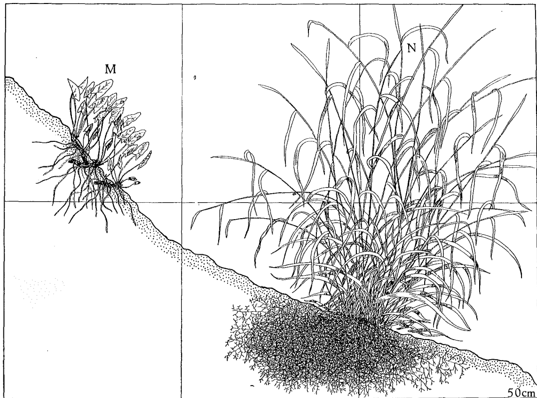
FIG. 14. — Profil de l'Arrhénathéraie.
