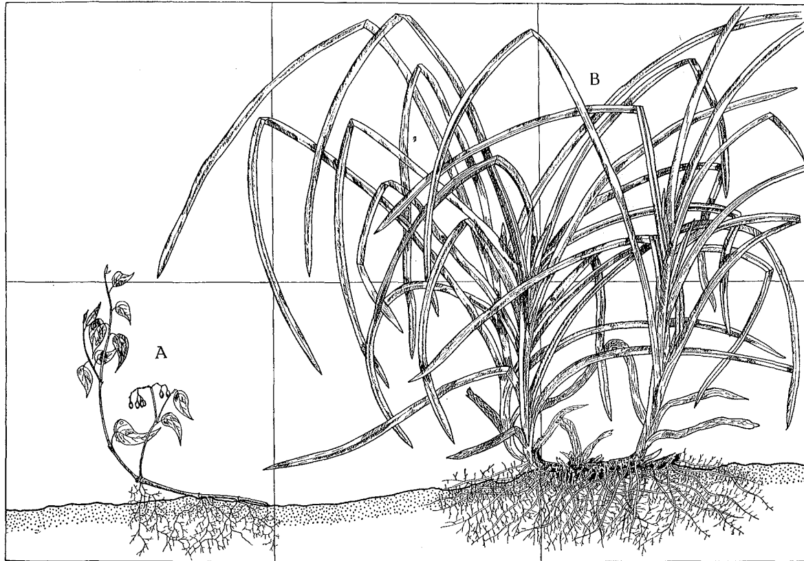
FIG. 6. — Profil du groupement fontinal. A = Solanum dulcamara L.; B = Carex pendula L.
