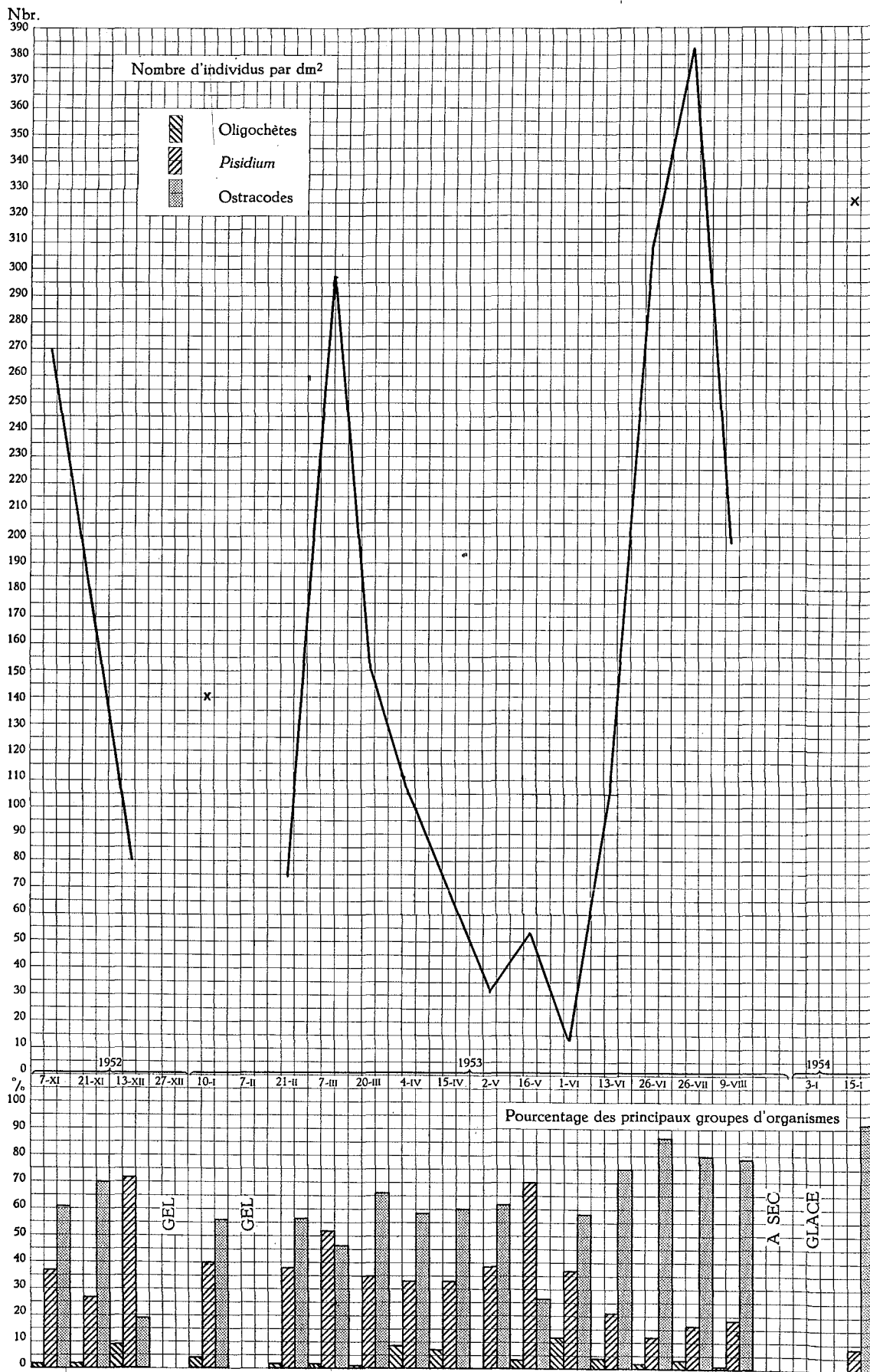
FIG. 18. — Variations saisonnières du benthos dans la zone à Glyceria aquatica (L.) WAHL.
