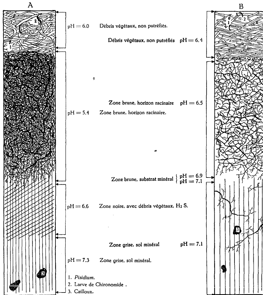
FIG. 7. — Coupes du fond des zones à carex et à glycéries. (S. JACQUEMART, 1955, fig. 1.)
