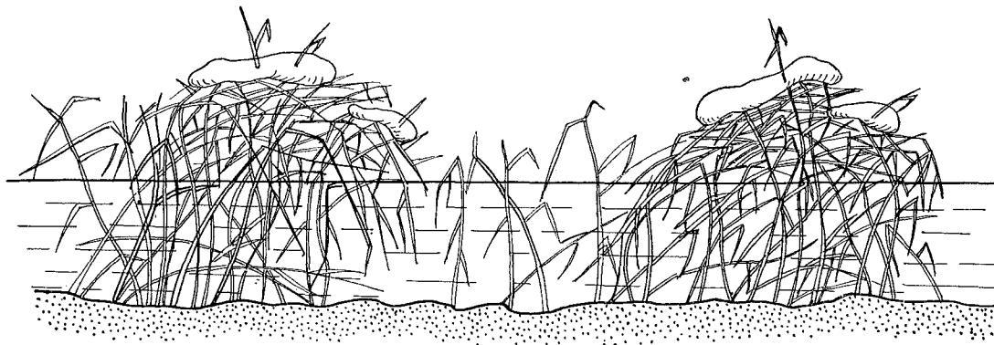
FIG. 15. — Schéma des hibernacula réalisés par les glycéries sèches (novembre-janvier).
