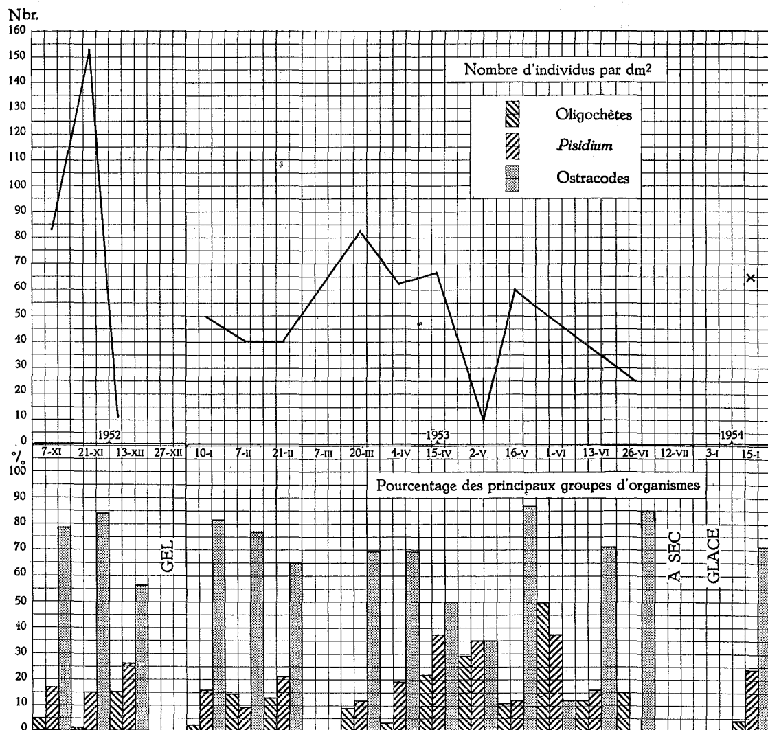
FIG. 19. — Variations saisonnières du benthos dans la zone à carex.
