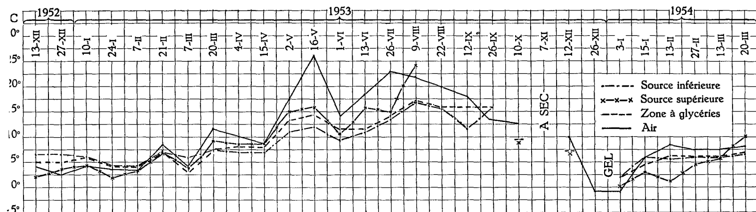
FIG. 4. — Courbes annuelles des températures des sources inférieure et supérieure, de la zone à glycéries et de l'air.
