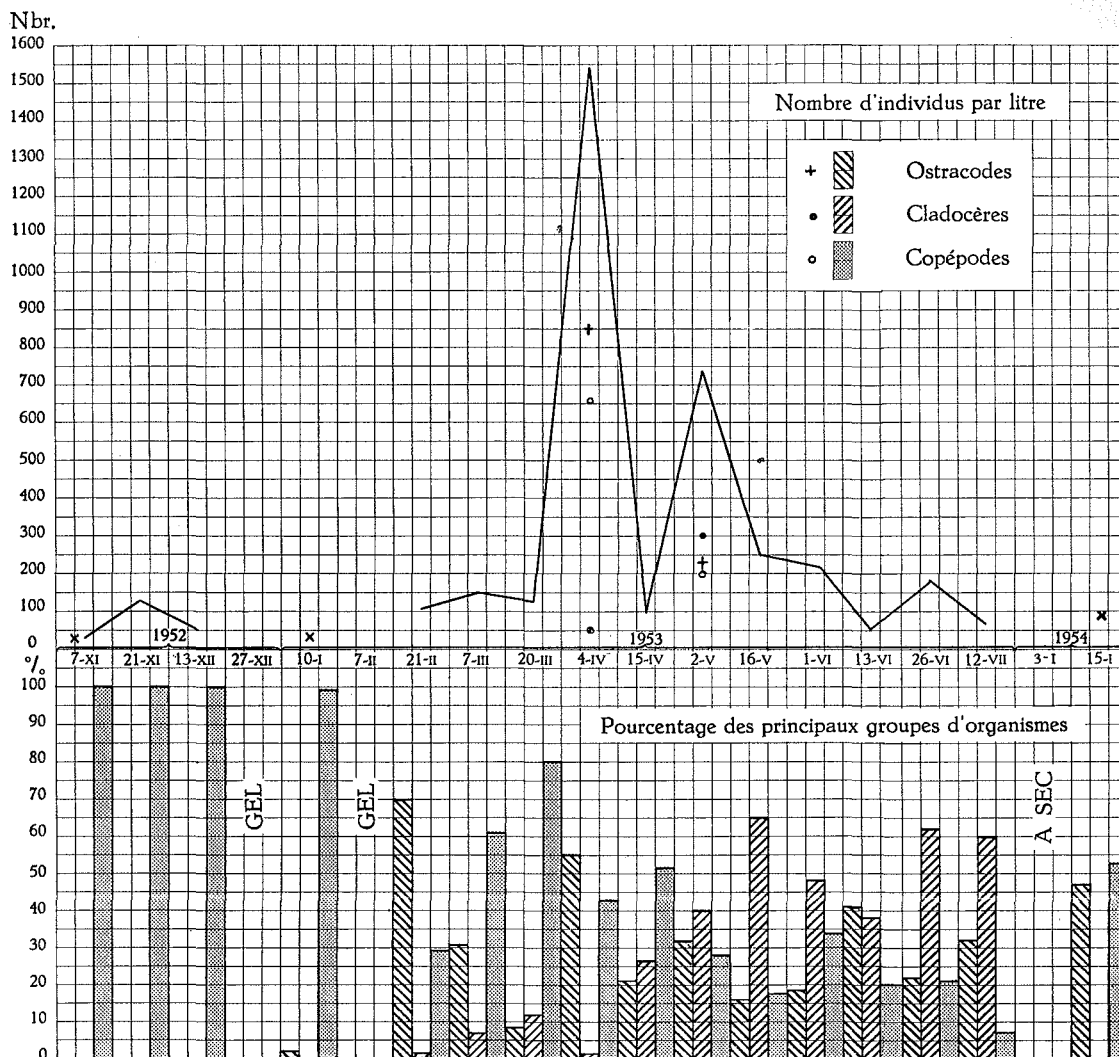
FIG. 17. — Variations saisonnières du plancton dans la zone à carex.
