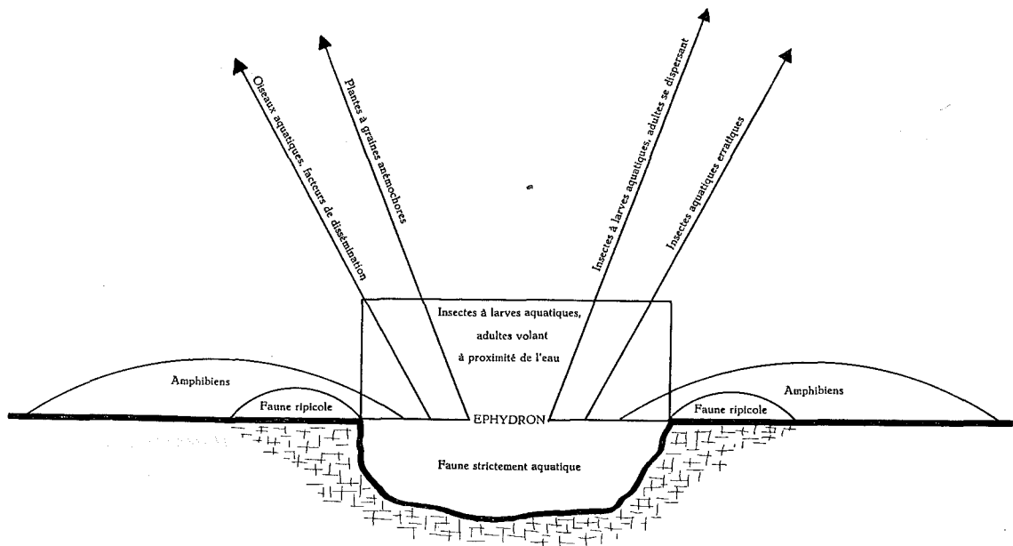
FIG. 20. — Schéma du rôle d'une mare dans la distribution des organismes.
