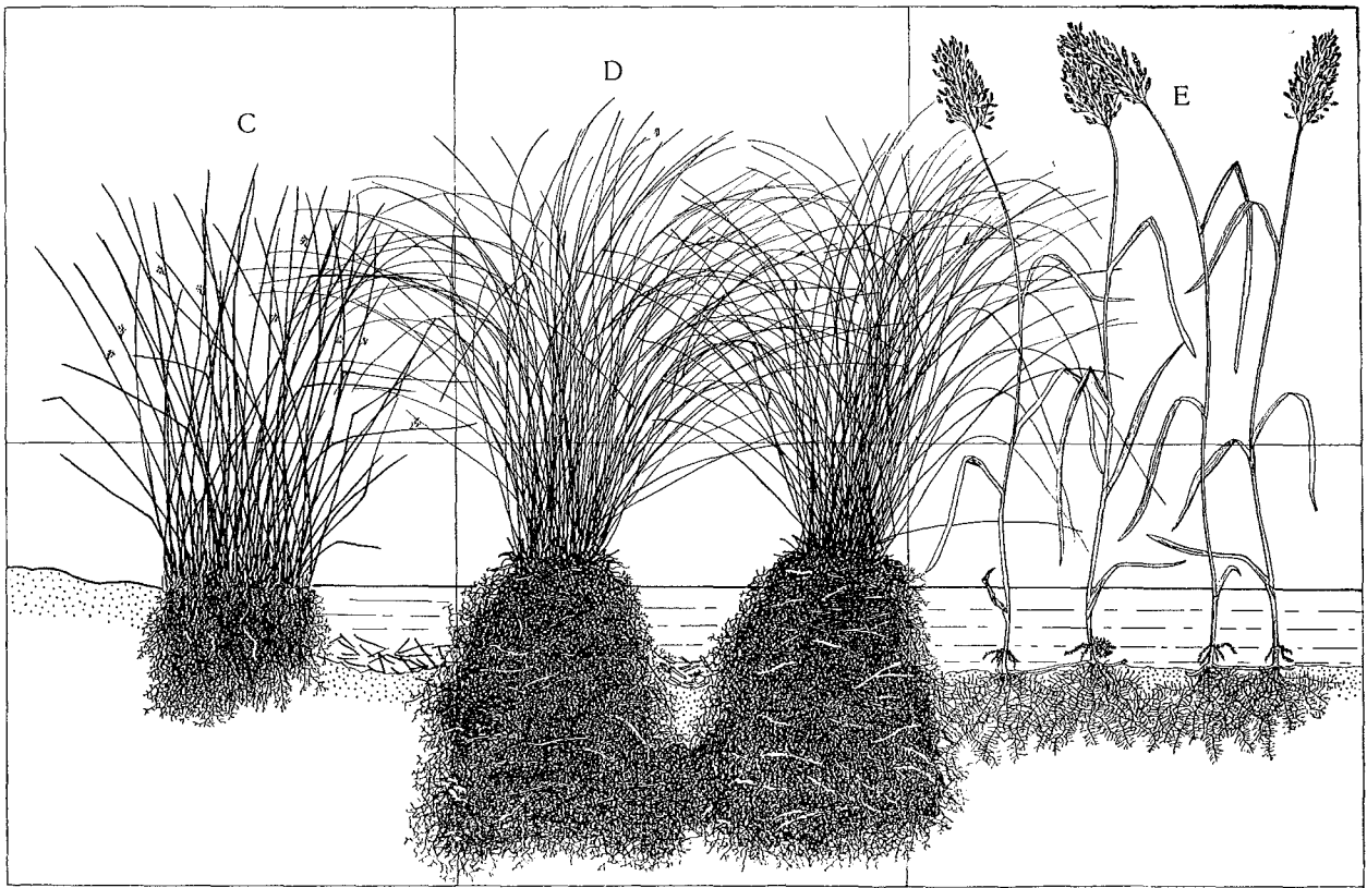
FIG. 8. — Profil des zones à juncs, carex et glycéries.
