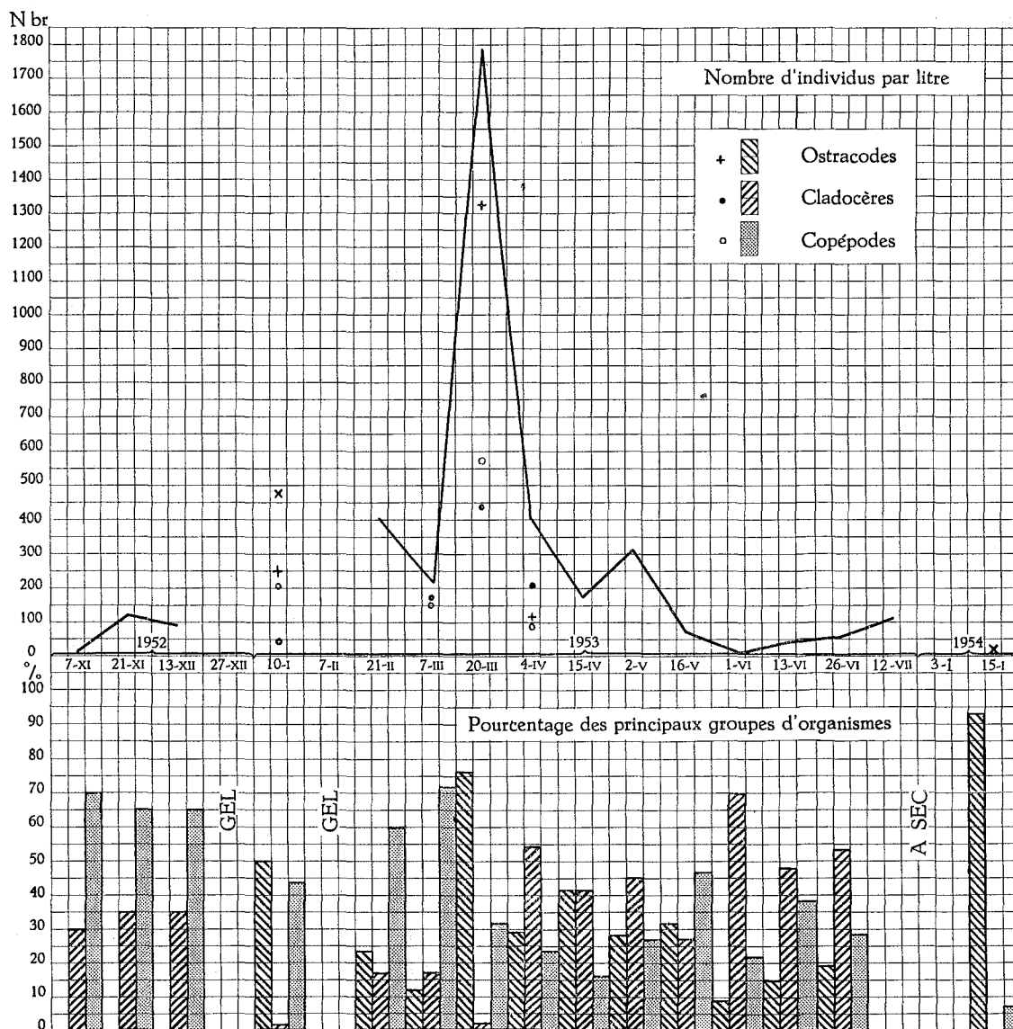
FIG. 16. — Variations saisonnières du plancton dans la zone à glycéries.
