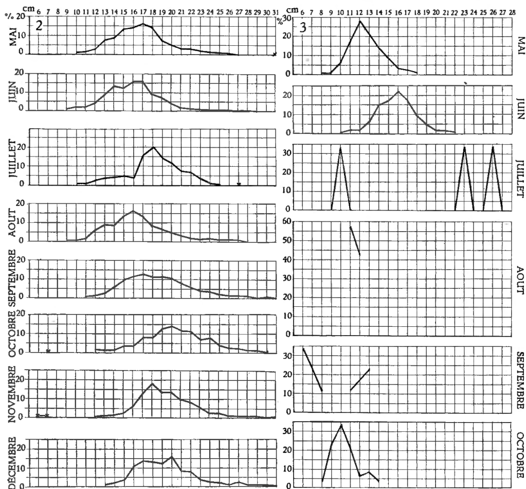
Fréquence de la taille en cm de : Fig. 2. — Limanda limanda (LINNÉ, 1758). Fig. 3. — Trigla lucerna (LINNÉ, 1758).
