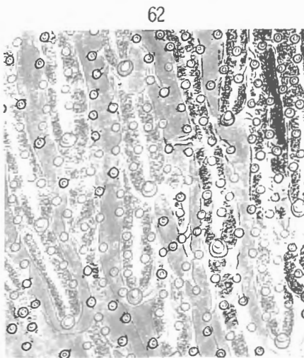
FIG. 62-63. — Mopalia heathii Pilsbry, 1898. Aesthètes. \times 260 . FIG. 62. — Région médiane. FIG. 63. — Région latérale.
